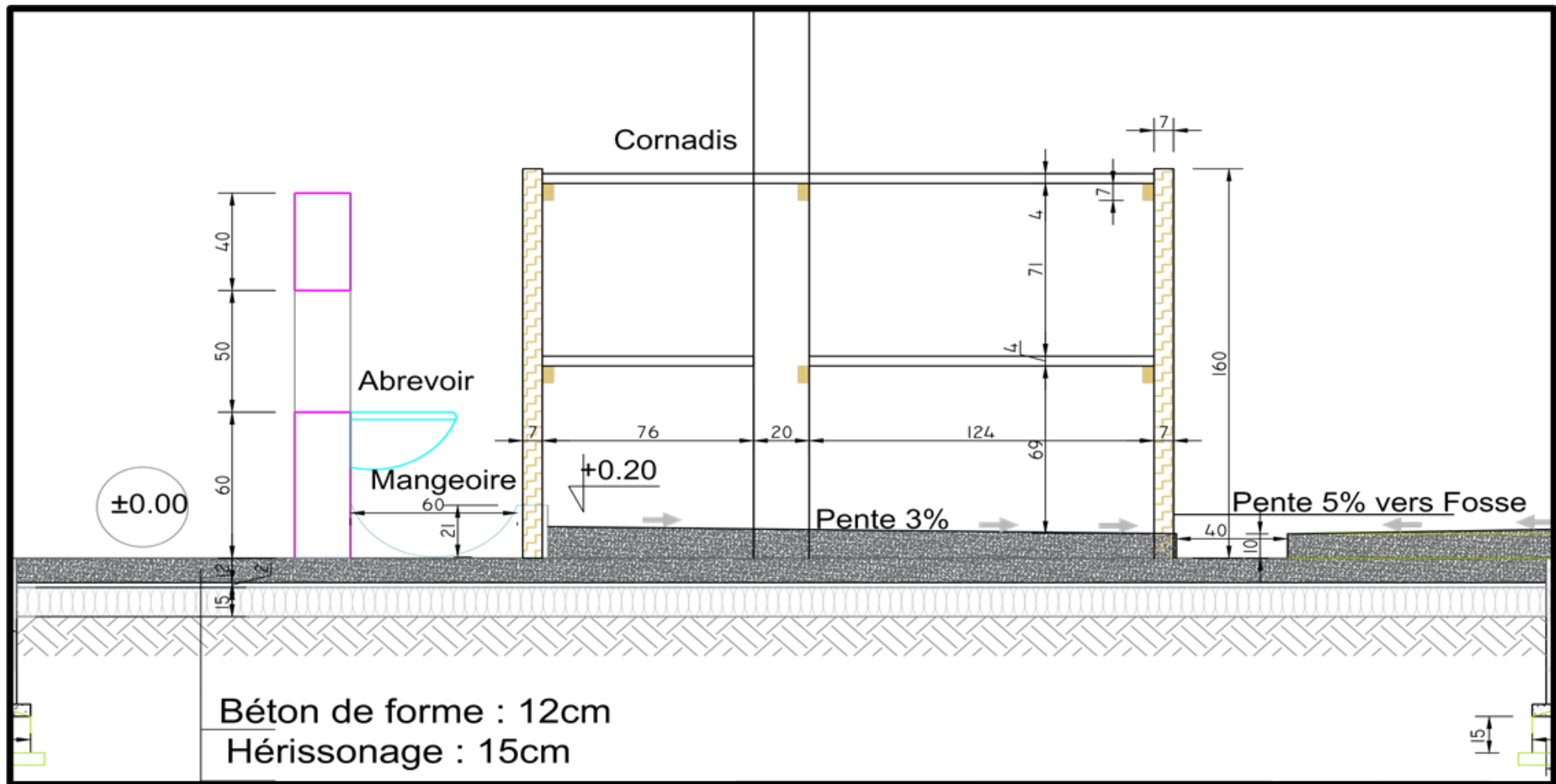
Annexe 01 : Plan type de dallage, mangeoire avec abreuvoir Coupe suivant la largeur d'étable (lot 1, lot 2, lot 3 et lot 4) :
